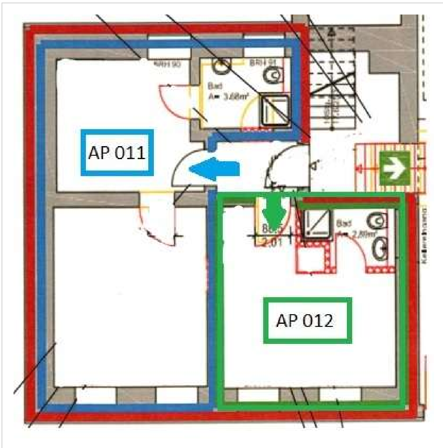
Grundriss WE1
